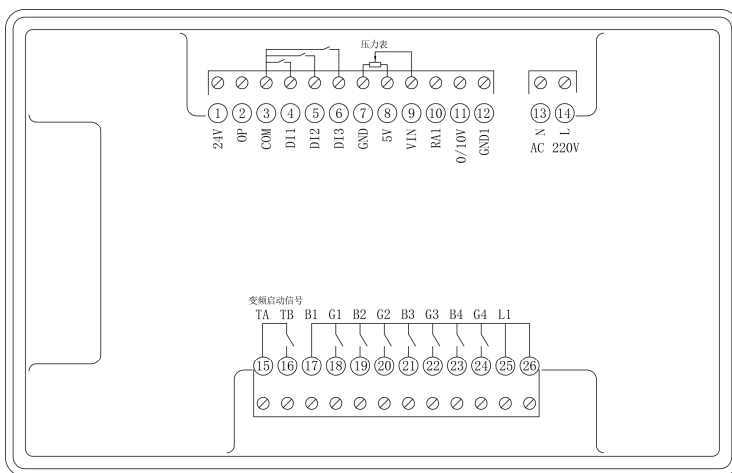
控制器接线端子示意图
