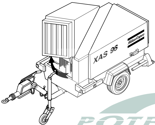
Fig. 2.1 Vista general del modelo XAS96 Dd con la puerta abierta (la barra de remolque ajustable con frenos y la rueda directriz son opcionales)
