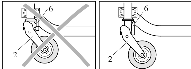
Fig. 3.3 Posición de aparcamiento de la rueda guía
