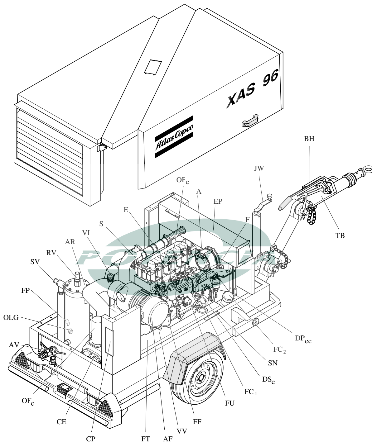
Fig. 2.2 Piezas principales del XAS96 Dd (la barra de remolque ajustable, la rueda guía, los frenos y la señalización de tráfico son opcionales)
