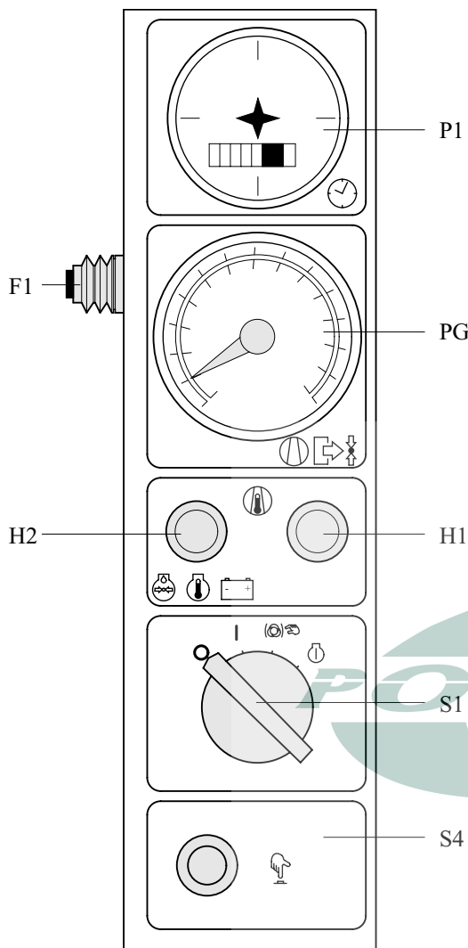
Fig. 3.10 Panel de operación
