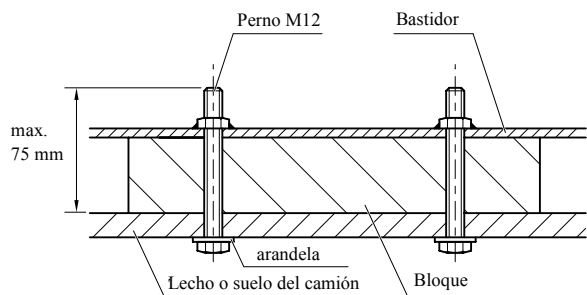
Fig. 8.3 Sección transversal
