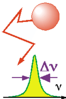
Abbildung 1.34: Bewegungsprozess erzeugen Relaxation.
