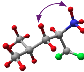
Abbildung 1.28: Prinzip einer Strukturbestimmung mit NMR.
