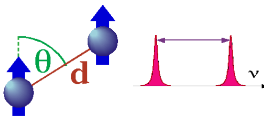
Abbildung 1.14: Die magnetische Dipol-Dipol Wechselwirkung spaltet die Resonanzlinien auf.
