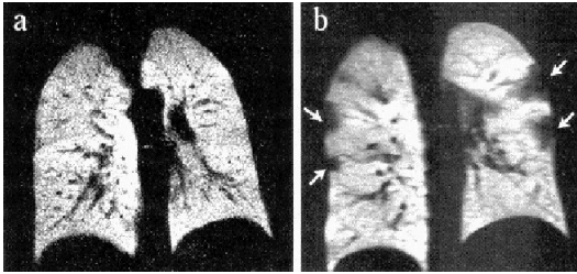
Abbildung 1.23: ^3\text{He} Bild einer gesunden Lunge (links) und einer Raucherlunge (rechts).
