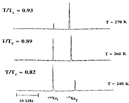
Abbildung 1.30: ^{129}\text{Xe} NMR von Gas und Flüssigkeit.
