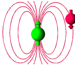
Abbildung 1.25: Wechselwirkung zwischen magnetischen Dipolen.
