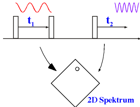
Abbildung 1.32: Prinzip der zweidimensionalen Spektroskopie.
