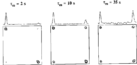
Abbildung 1.31: 2D Austauschspektroskopie an einem Xe Zweiphasensystem.
