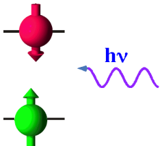
Abbildung 1.1: Resonante Anregung von Spin-Übergängen
