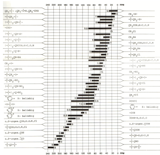
Abbildung 1.17: Übersicht über die wichtigsten Bereiche der chemischen Verschiebung von 13 C.
