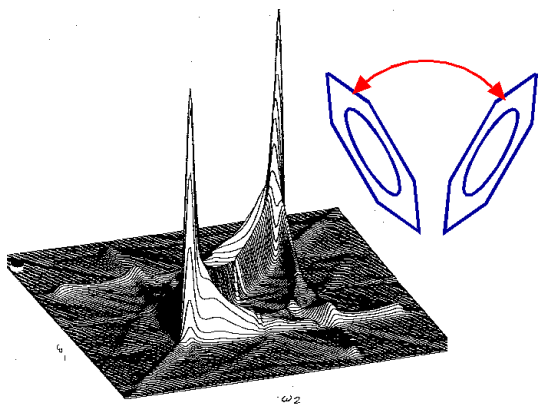
Abbildung 1.33: 2D Austausch-NMR an deuteriertem Benzol.
