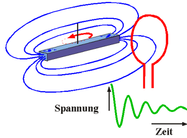
Abbildung 1.6: Präzedierende Magnetisierung erzeugt in der Detektorspule eine Induktionsspannung.
