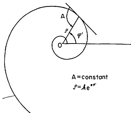
Fig. 1—The equiangular spiral.
