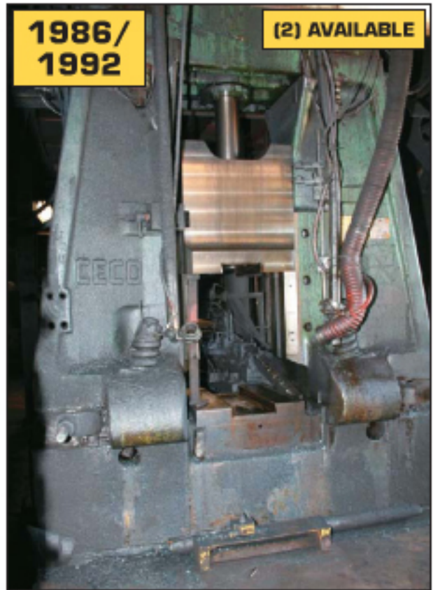
Chambersburg/Ceco Die Forger, MDL 14
