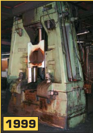
1999 Chambersburg/Ceco Die Forger, Mdl. 23
