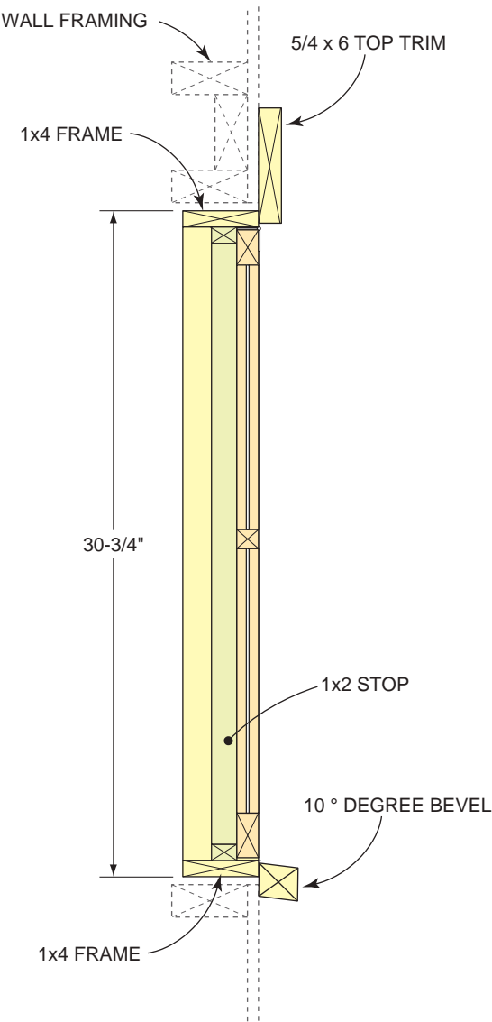
SECTION A-A
