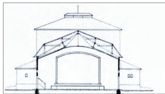
A színház metszete
