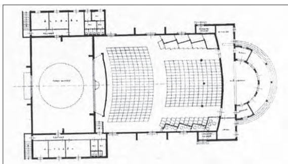
A színház alaprajza
