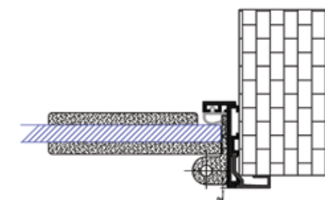
INSTALLAZIONE A MURO CON COPRIFILO GLASS TO GLASS INSTALLATION
