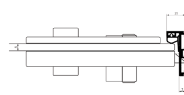
APPLICAZIONE CON SERRATURE 15100 15100 LOCK INSTALLATION
