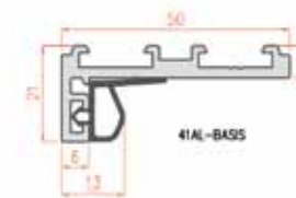
PROFILO A STIPITE, 41 AL BASIS
