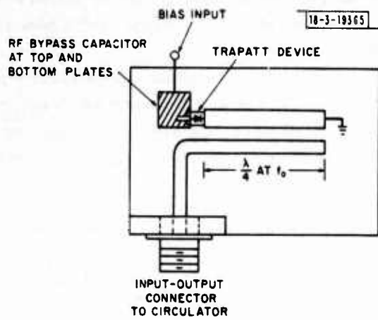
Fig. VI-6. Coupled-line amplifier.
