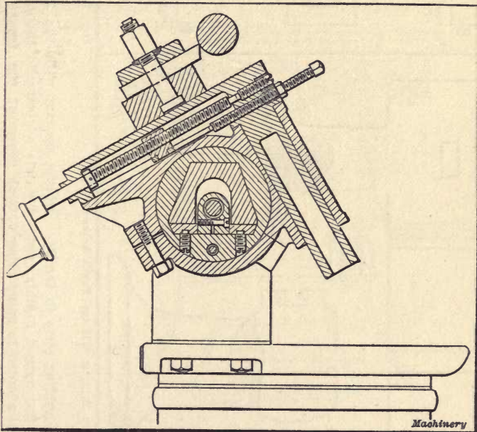
Fig. 28. The Pittler Trapezoidal Bed used by the Leipziger Werkzeugmaschinenfabrik, Leipzig-Wahren, Germany
