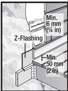
Figure 10 Drip Edge
