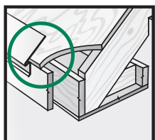
Figure 10 Drip Edge
