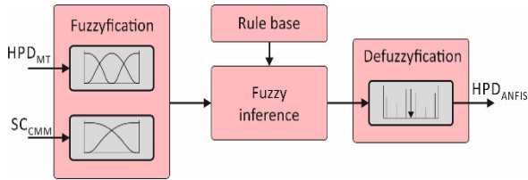
Fig. 5. ANFIS scheme.
