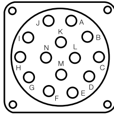
MOTOR MS3102E-20-27P
