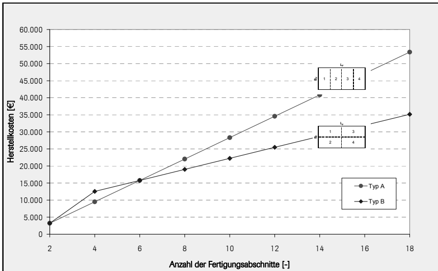
Abb. 2-25 Herstellkosten für Typ A und Typ B – Vergleich
