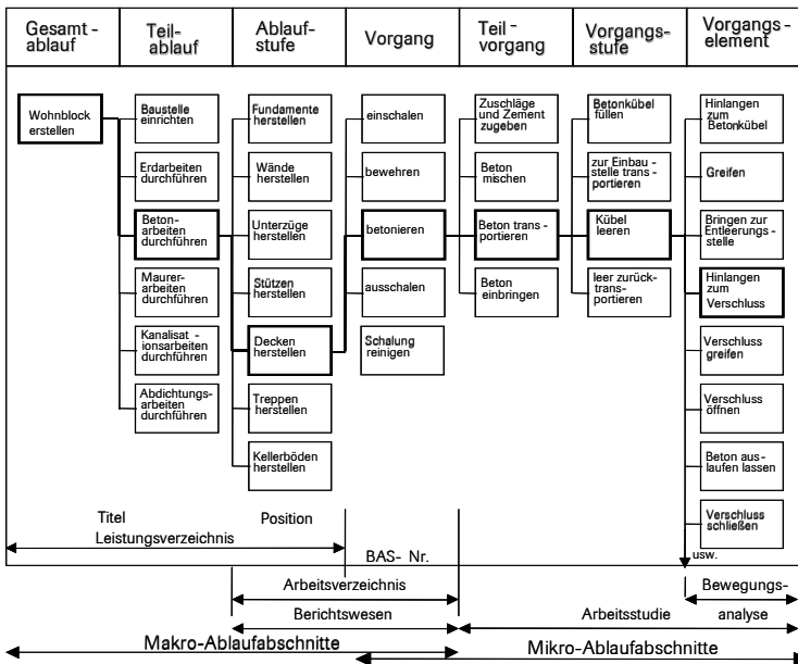
Abb. 2-15 Unterteilung eines Bauwerks in Ablaufabschnitte 57)
