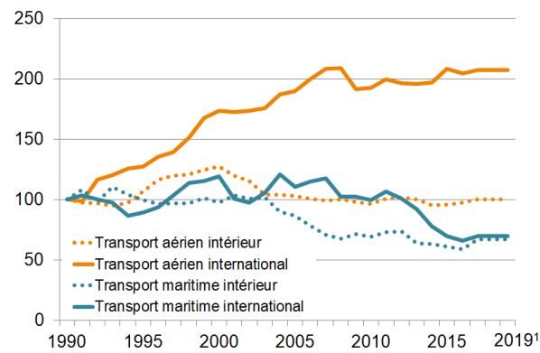
Figure D2.1-7 Évolution des émissions de GES, intérieures et internationales du transport aérien et du transport maritime
