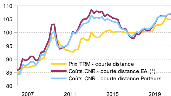
Figure B2.2-3 Prix et TRM courte distance
