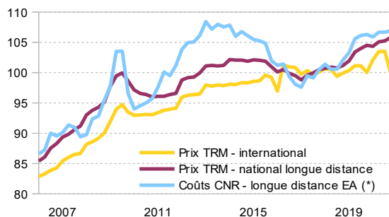
Figure B2.2-2 Prix et coûts TRM longue distance
