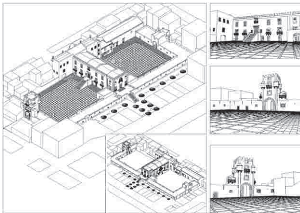
Assonometrie Palazzo Butera
