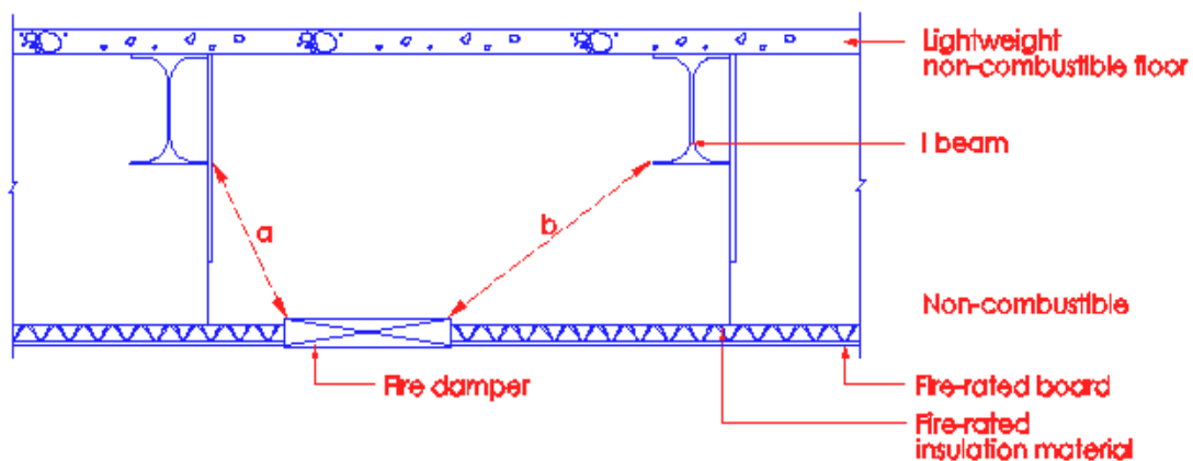
Diagram 7.1.1(ii)
