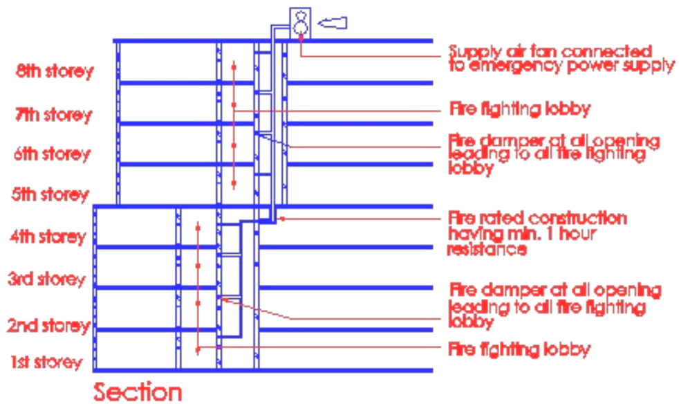
Diagram 7.1.4(d)
