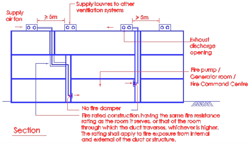
Diagram 7.1.5(b)
