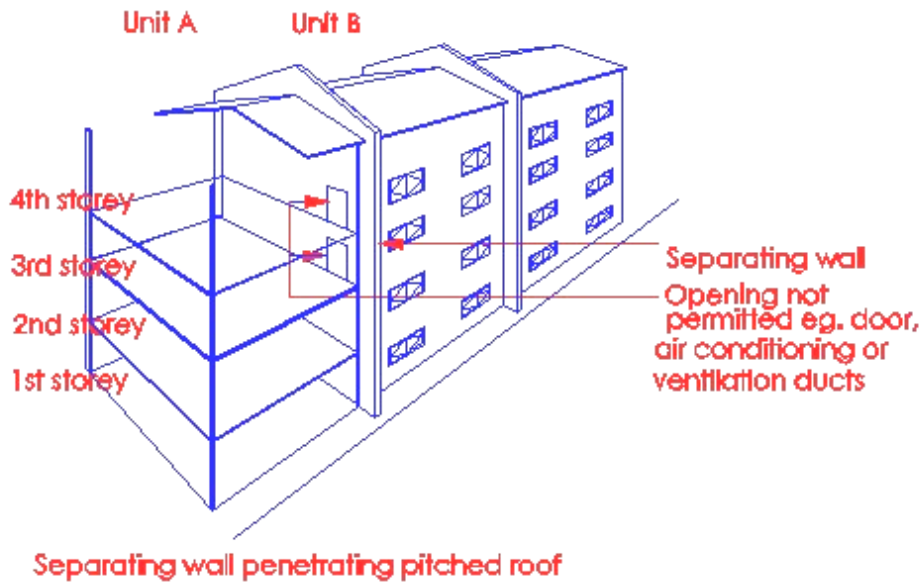
Diagram 7.1.1(g)
