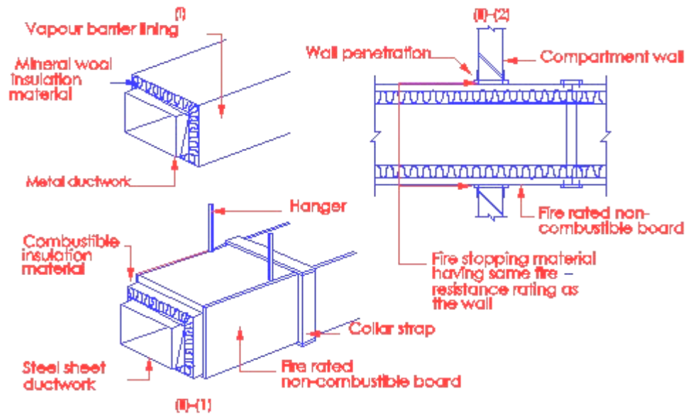
Diagram 7.1.1(b)
