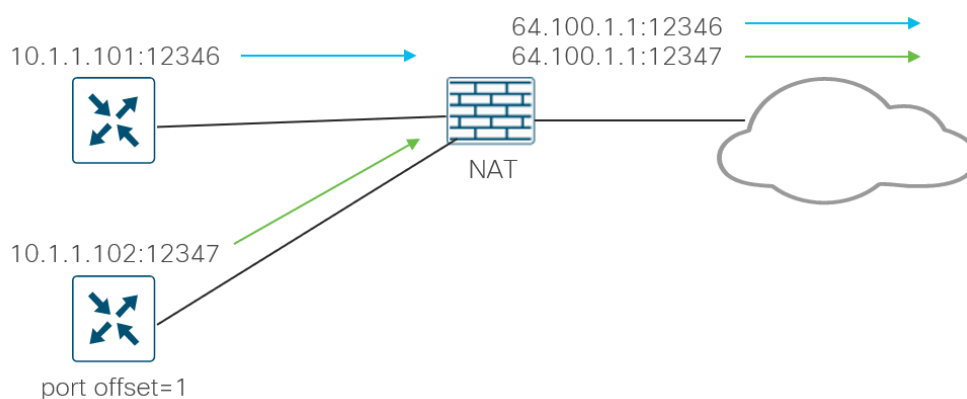
Figure 37. Wan Edge port offset
