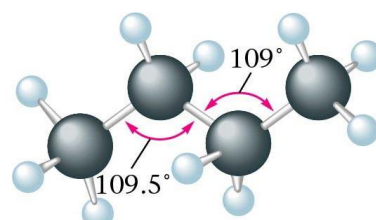
(b) Butane
