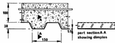
Fig. 2.8 Composite slab.
