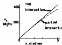
Fig. 2.18 Longitudinal shear force per unit length.
