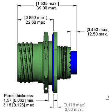
Fig. 2 Jam nut receptacles
