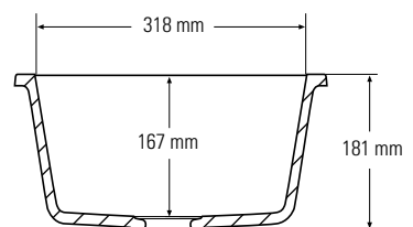
Querschnitt Seitenansicht
