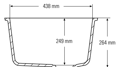
Querschnitt Seitenansicht
