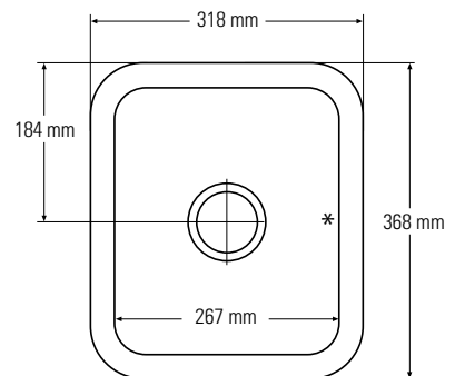
Ansicht von oben * Überlauf
