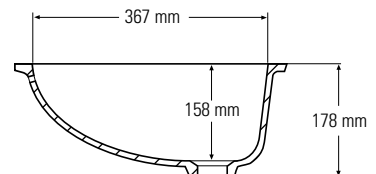
Querschnitt Seitenansicht
