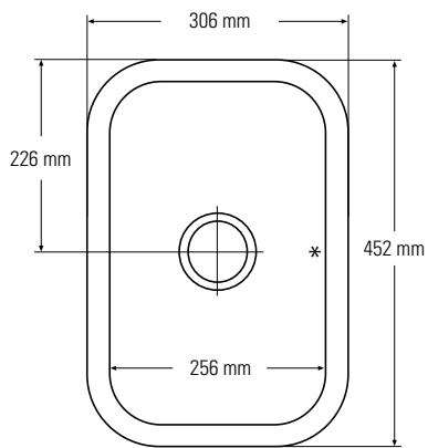
Ansicht von oben * Überlauf
