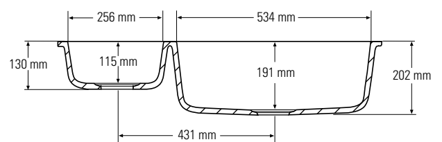
Querschnitt Seitenansicht
