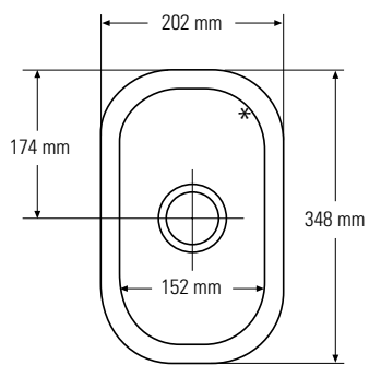
Ansicht von oben * Überlauf
