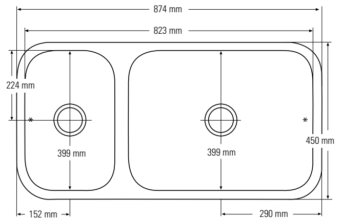
Ansicht von oben * Überlauf
