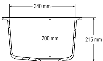
Querschnitt Seitenansicht
