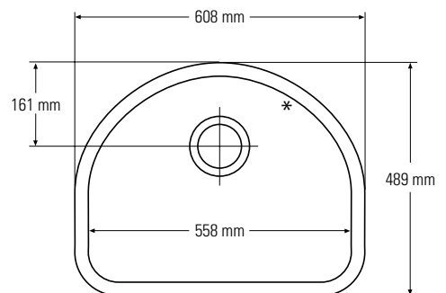
Ansicht von oben * Überlauf
