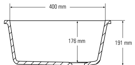
Querschnitt Seitenansicht
