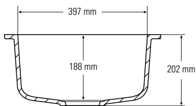
Querschnitt Seitenansicht
