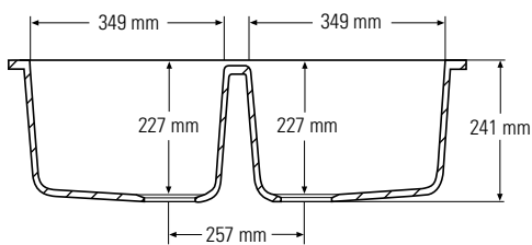
Querschnitt Seitenansicht
