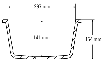
Querschnitt Seitenansicht
