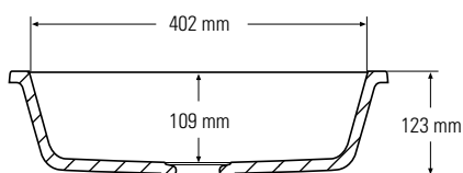
Querschnitt Seitenansicht
