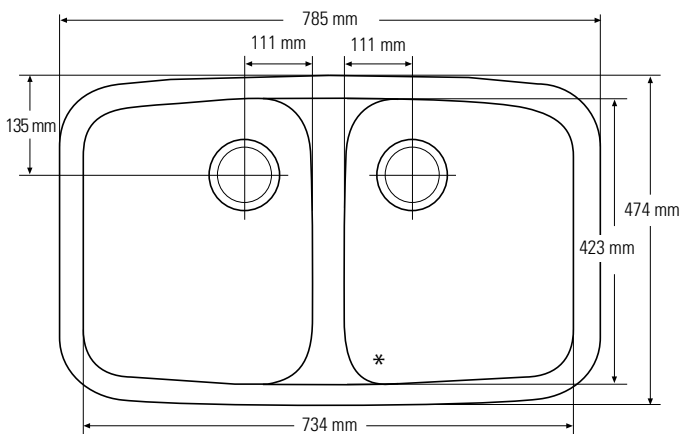
Ansicht von oben * Überlauf
