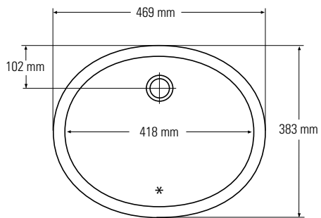
Ansicht von oben * Überlauf
