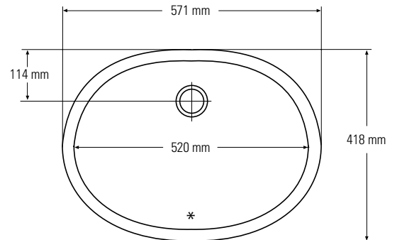
Ansicht von oben * Überlauf
