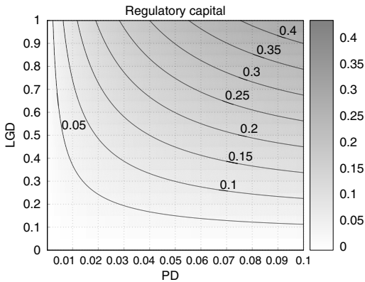
(b) RC: \varrho = 20\% , M=1 (contour)
