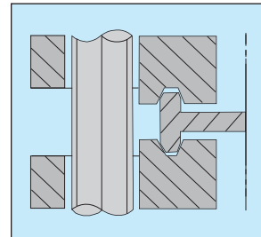
Junta Tipo RTJ Ciega
