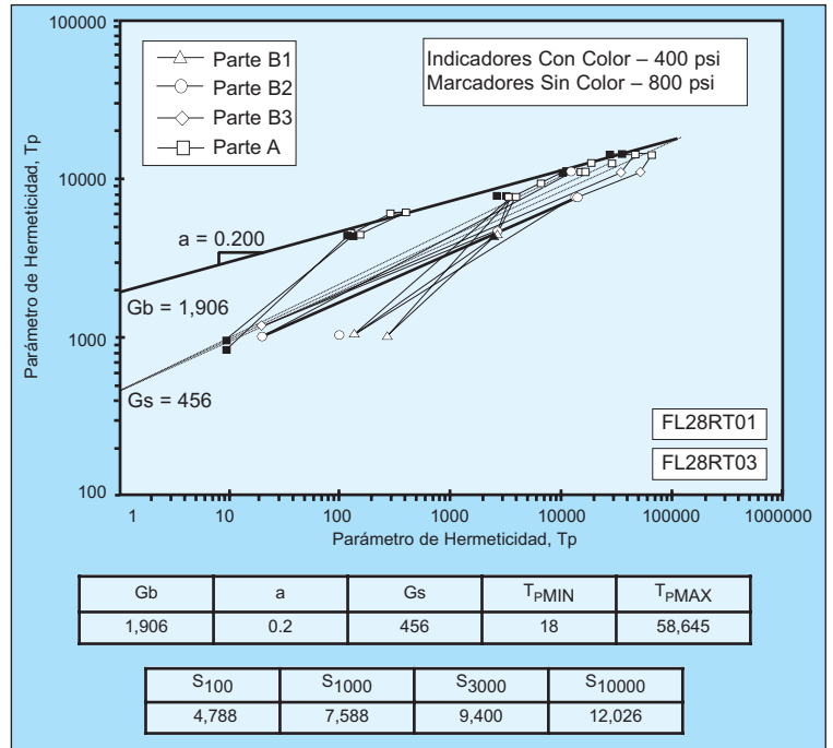
Caracterización del comportamiento de la Hermeticidad en Temperatura Ambiente (ROTT – por sus siglas en inglés). (Refiérase a la página 43 para el nuevo método para determinar los factores).
