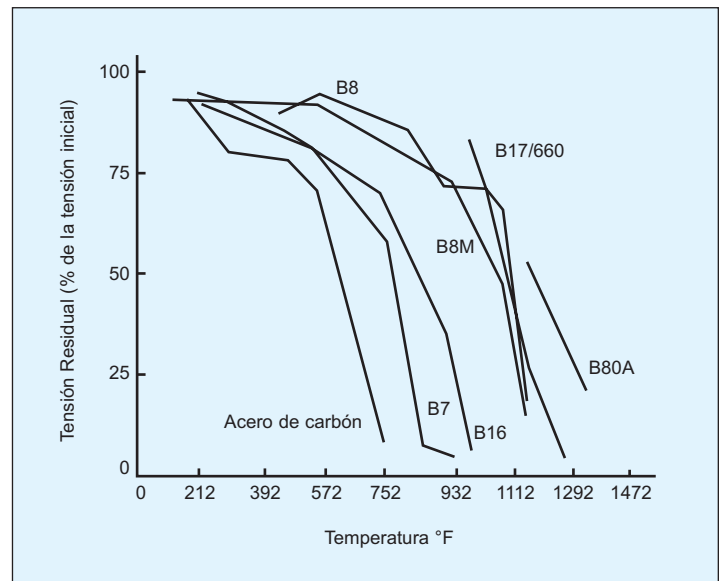
Comportamiento de relajación de la tensión de diversos tipos de tornillos mostrando el porcentaje de la tensión inicial retenida a la temperatura
