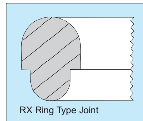
Junta Tipo RTJ de Transición
