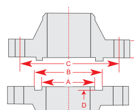
Lengüeta y Ranura
