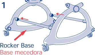
2 Straight Tubes 2 el tubo recto
