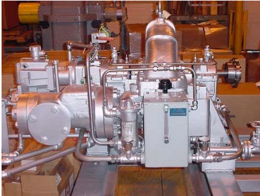
Turbina de vapor marca Coppus-Dresser Rand RLHA15 para accionamiento de bomba centrífuga horizontal instalada en la Refinería Salina Cruz Oaxaca ( 2005 )
