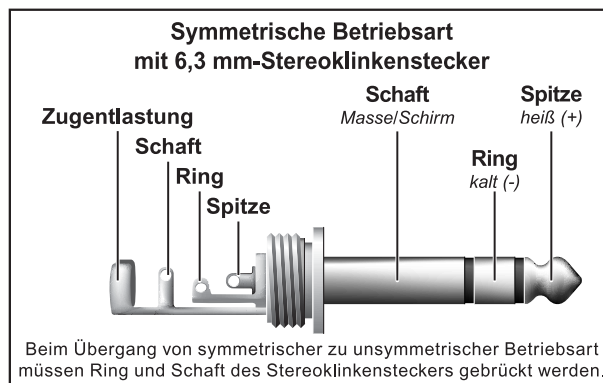
Abb. 4.4: 6,3 mm-Stereoklinkenstecker
