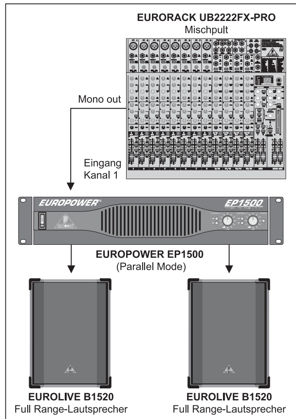
Abb. 3.3: Parallelbetrieb
