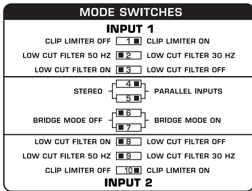
Abb. 3.4: DIP-Schalteneinstellungen für den Parallelbetrieb
