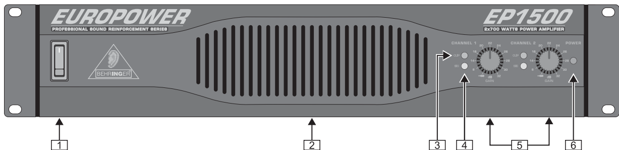
Abb. 2.1: Die frontseitigen Bedienungselemente
