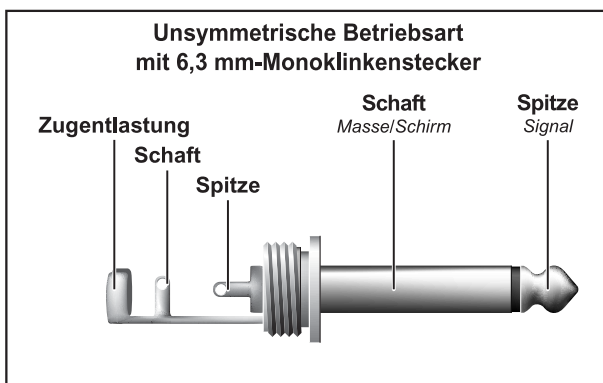
Abb. 4.3: 6,3 mm-Monoklinkenstecker
