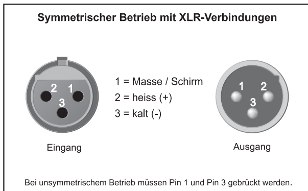
Abb. 4.2: XLR-Verbindungen
