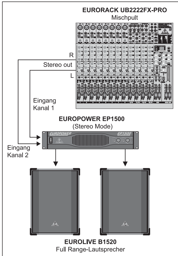
Abb. 3.1: Zweikanalbetrieb
