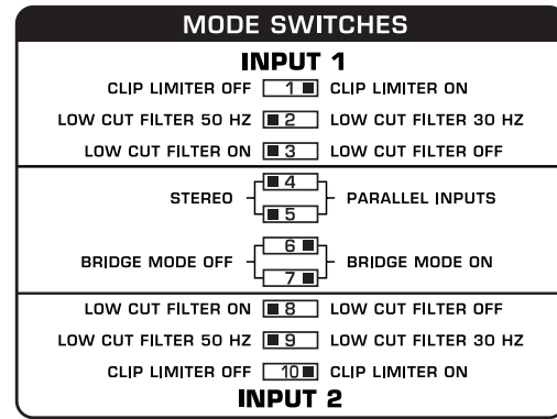
Abb. 3.6: DIP-Schalteneinstellungen für den Monobrückenbetrieb
