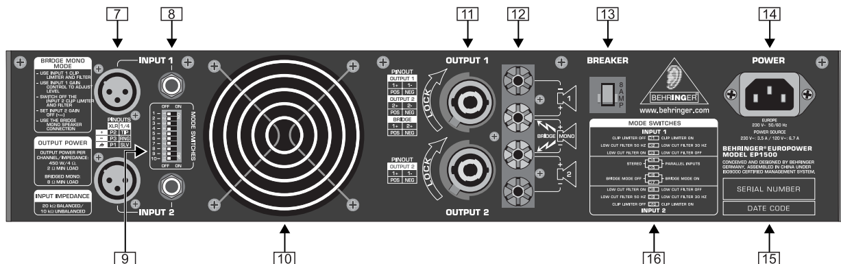
Abb. 2.2: Die rückseitigen Bedienungselemente und Anschlüsse
