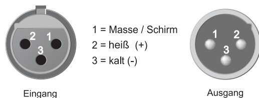
Abb. 8.1: XLR-Verbindungen
