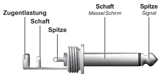
Abb. 8.2: 6,3 mm-Monoklinkenstecker
