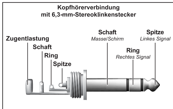
Abb. 8.4: Kopfhörer-Stereoklinkenstecker
