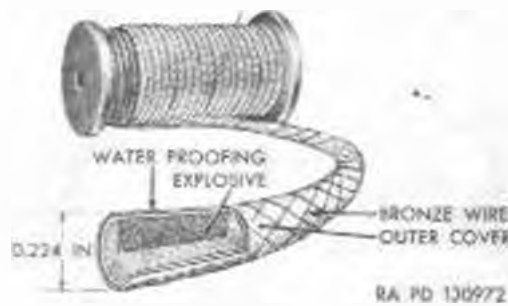
Figure 23. Cord, detonating (PETN) (fuze, primacord).
