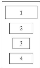
BoxLayout (vertical)
