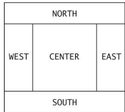
BorderLayout
