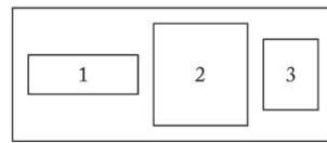
BoxLayout (horizontal)
