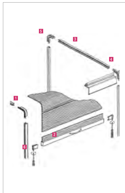
Esquema de armado y componentes
