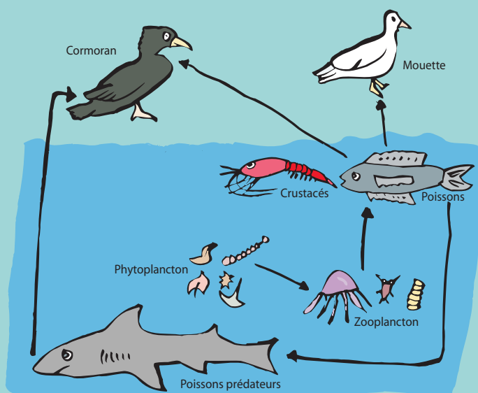
La chaîne alimentaire marine
