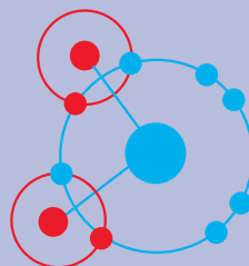
Structure de la molécule d'eau
