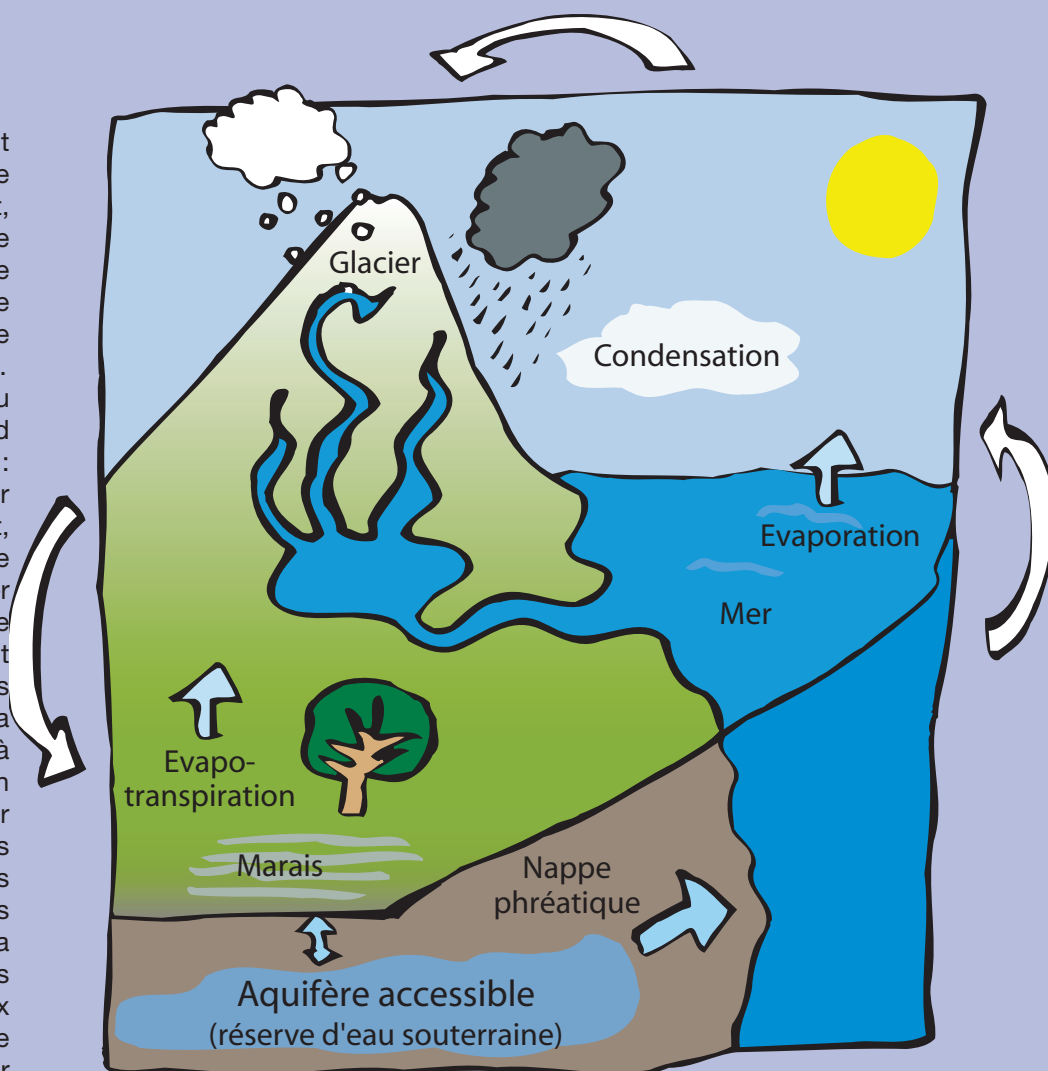
Le cycle de l'eau
