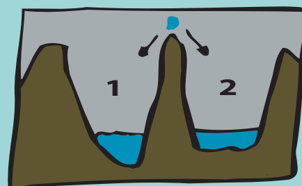
Structure de deux bassins-versants
