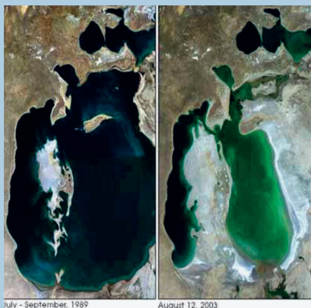
Vue satellite de l'assèchement de la mer d'Aral, Asie centrale (1989-2003)
