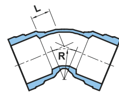
Socket / Socket
