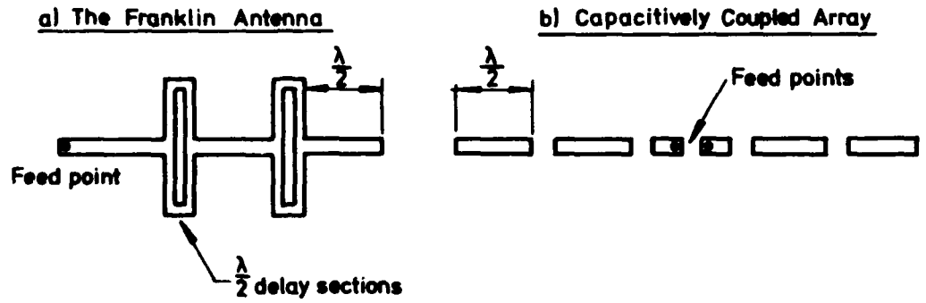
FIG. 2.8. COLINEAR DIPOLE ARRAYS
