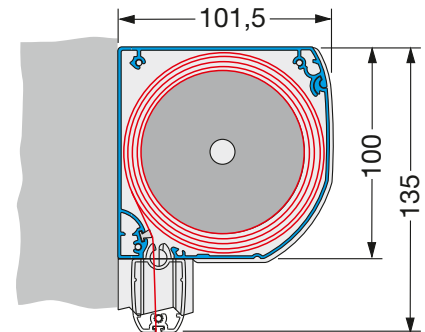
MICRO 1000/1000 (Z)
