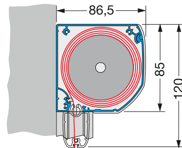
MICRO 850/850 (Z)
