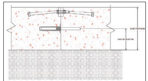
Step 4: Place Taper Dowel and Pour Other Side.
