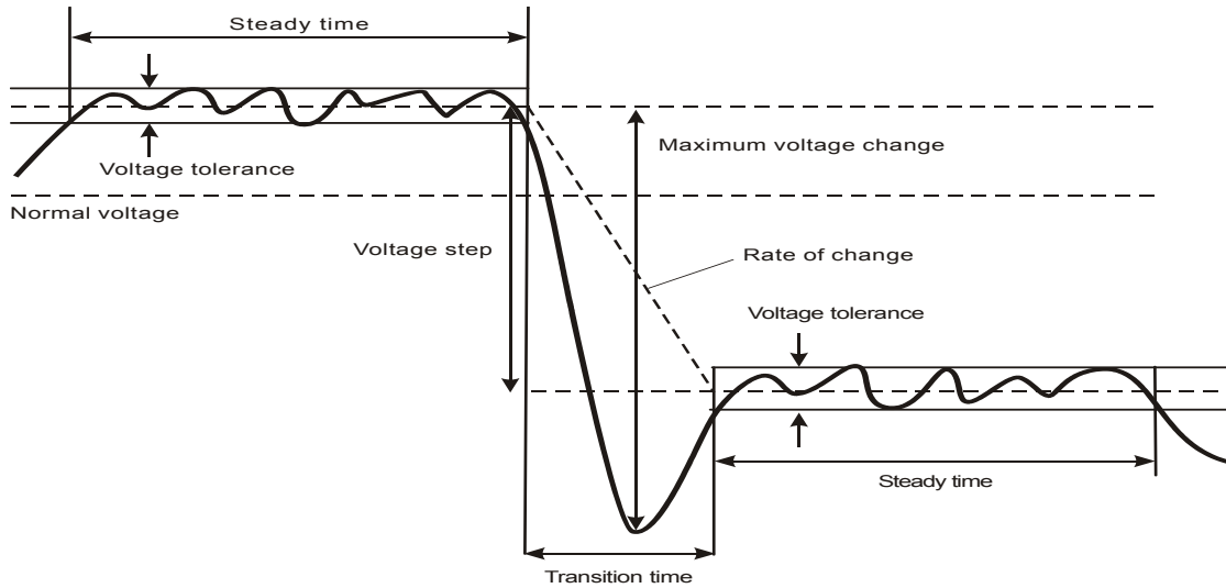
Figura 9-4. Características de un cambio rápido de tensión
