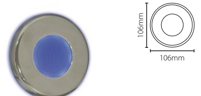
Proximity lecteur Marin - chrome
