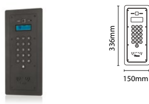
Net2 Entry - Platine Standard, Pose en encastré
