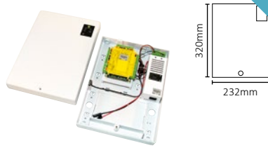
Net2 classic contrôleur 1 porte - Alim. 12V 2A, Coffret ABS
