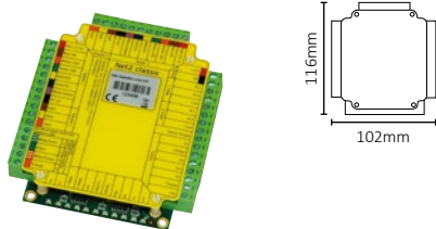
Net2 classic contrôleur 1 porte
