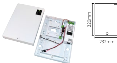
Paxton alimentation 12V 2A DC - coffret ABS
