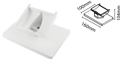
Net2 Entry - Support de bureau moniteur
