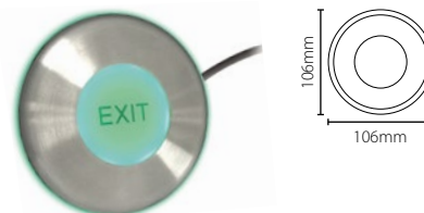
Paxton Bouton de sortie Marin
