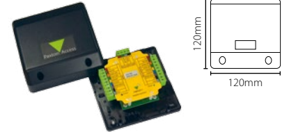
Proximity Interface Mains Libres - boîtier ABS
