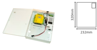
Net2 classic contrôleur 1 porte - Alim. 12V 2A, Coffret métal
