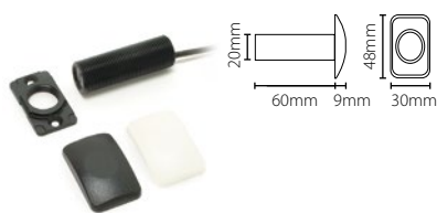
Proximity lecteur anti-vandale
