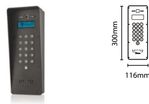
Net2 Entry - Platine Standard, Pose en saillie avec visière anti-pluie
