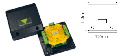
Proximity Interface Mains Libres - boîtier ABS
