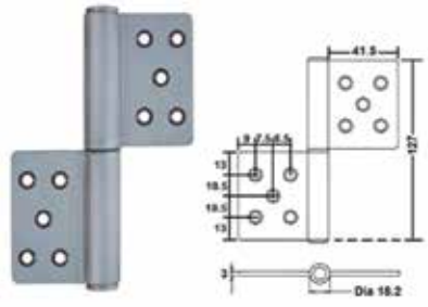
A01-028 125 x 102 x 3mm SUS 304 Stainless Steel Flag Hinge
