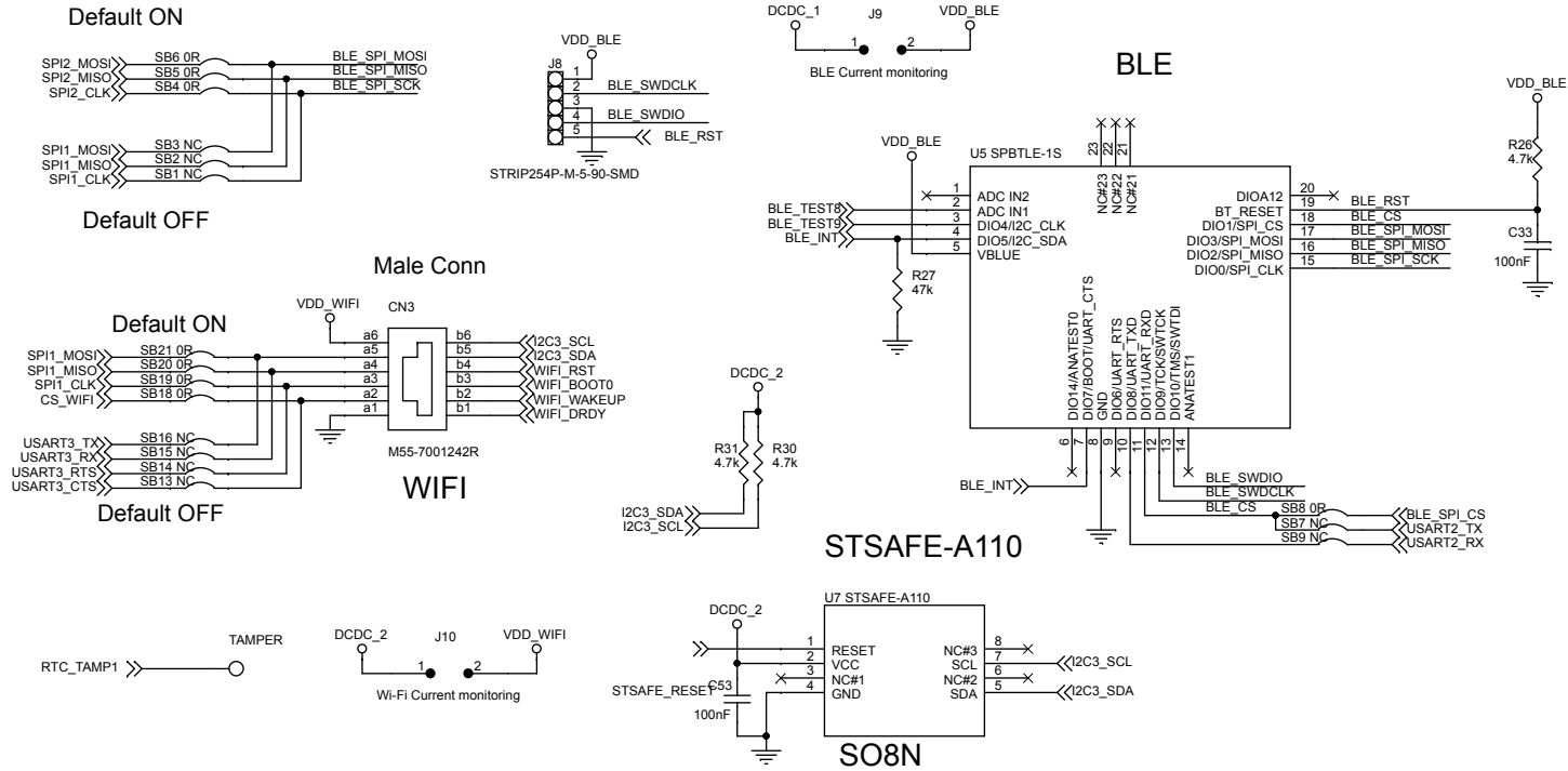
Figure 36. STEVAL-STWINKT1 schematic - BLE, Wi-Fi, STSAFE-A110
