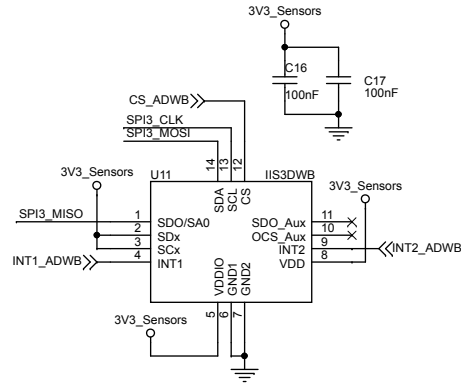
Vibrometer
