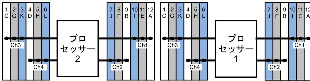
ProLiant DL360 Gen9 サーバーのプロセッサとメモリ スロットのレイアウト
