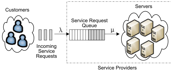
Fig. 2. The M/M/m queuing model.
