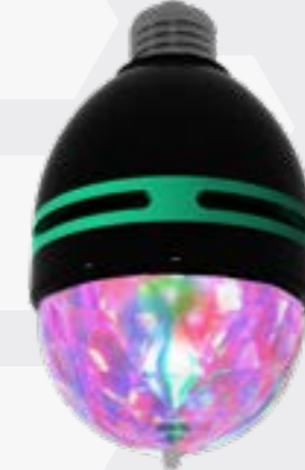
8717278 . 86349 . 8 E27 Fitting - 85/230V AC H.150 x Ø. 80 mm.
