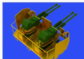
BIG5325 USS MISSOURI ČÁST I. 1/200 TRUMPETER
