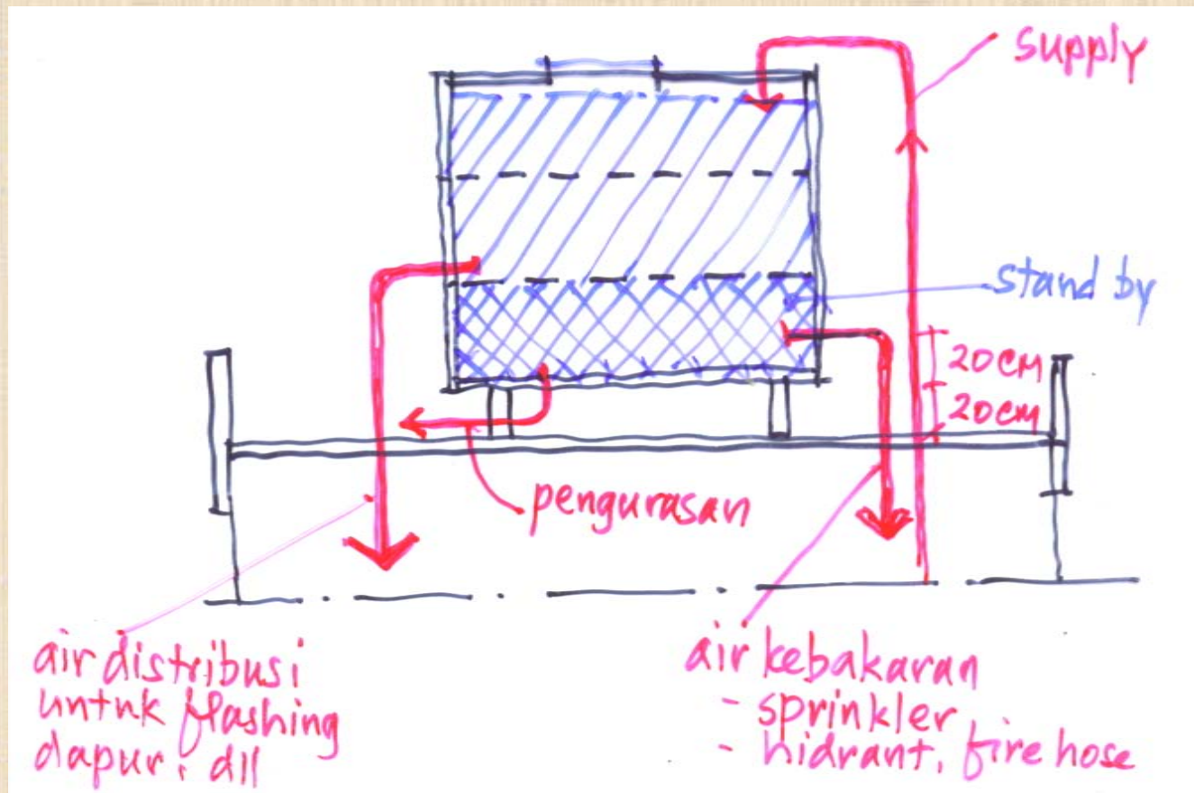
Pembagian air pada tangki atap
