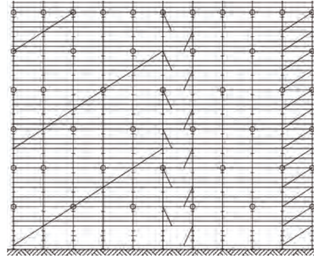
Fig. 93: Módulo de anclaje 8,00 m., distribuidos a tresbolillo cada 4,00 m. en vertical
