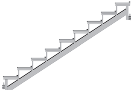
Viga escalera 500 LW , de 9 peldaños ref. 2639.009 Viga escalera 500 LW , de 5 peldaños ref. 2639.004
