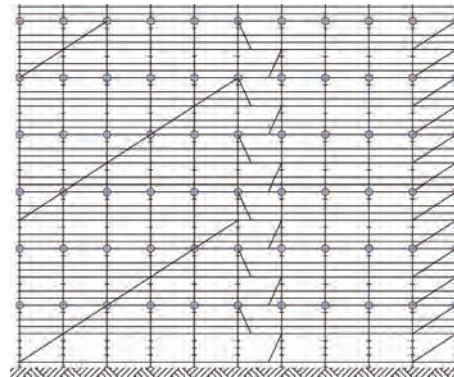
Fig. 94: Módulo de anclaje 4,00 m.
