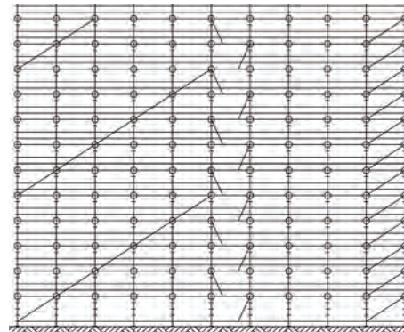
Fig. 95: Módulo de anclaje 2,00 m.
