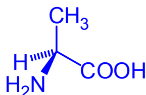
(+)-alanine ( L-alanine S-alanine
