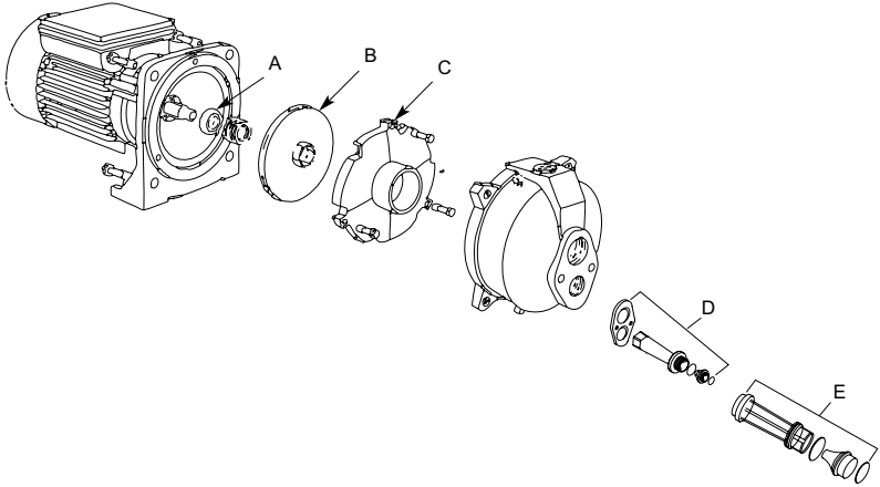
Figura 13: ilustración de las piezas de reparación para las bombas de chorro convertibles
