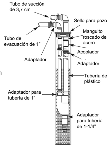
Figura 3: eyector para pozo profundo
