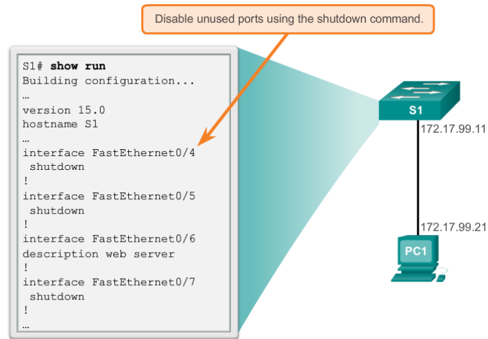
Fig. 2.8 Port yang Tidak Terpakai Pada Switch
