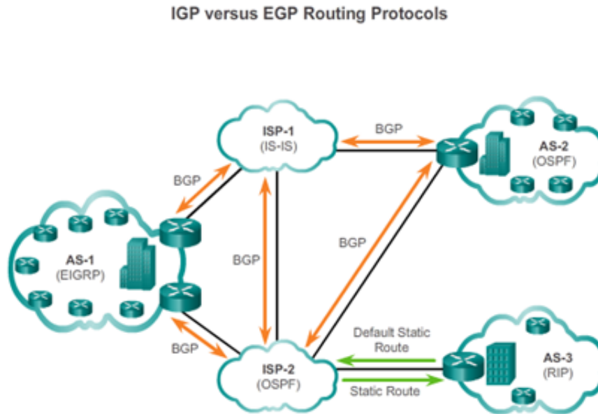
Fig. 7.9 Protokol Routing IGP dan EGP
