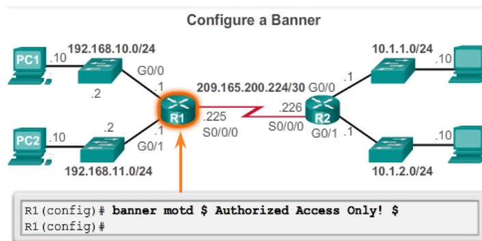
Fig. 4.6 Konfigurasi akses manajemen
