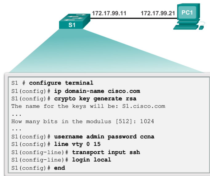
Fig. 2.5 Contoh Konfigurasi SSH
