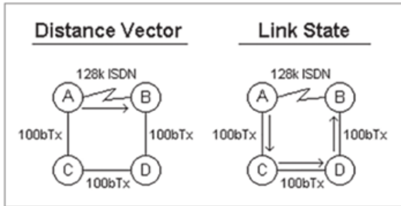
Fig. 7.21 Perbandingan Distance Vector dan Link State
