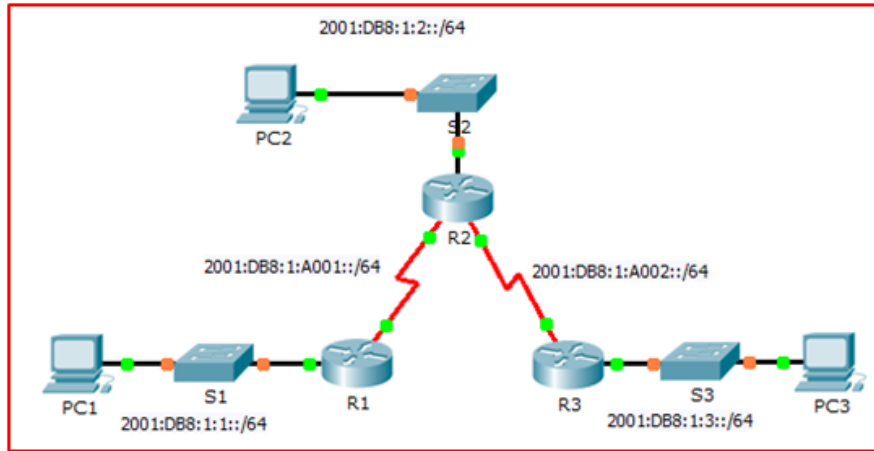
Fig. 6.9 Konfigurasi IPv6 Static Routing Pada Topology Jaringan
