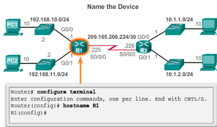
Fig. 4.5 Konfigurasi nama perangkat
