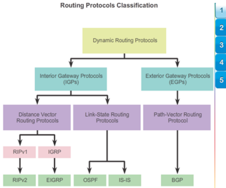
Fig. 7.7 Klasifikasi Protokol Routing
