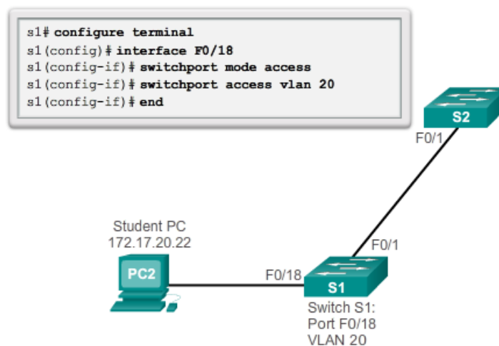
Fig. 3.10 Contoh Konfigurasi Port VLANs
