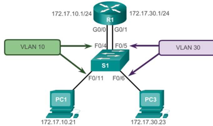
Fig. 5.1 Topologi Inter-VLAN
