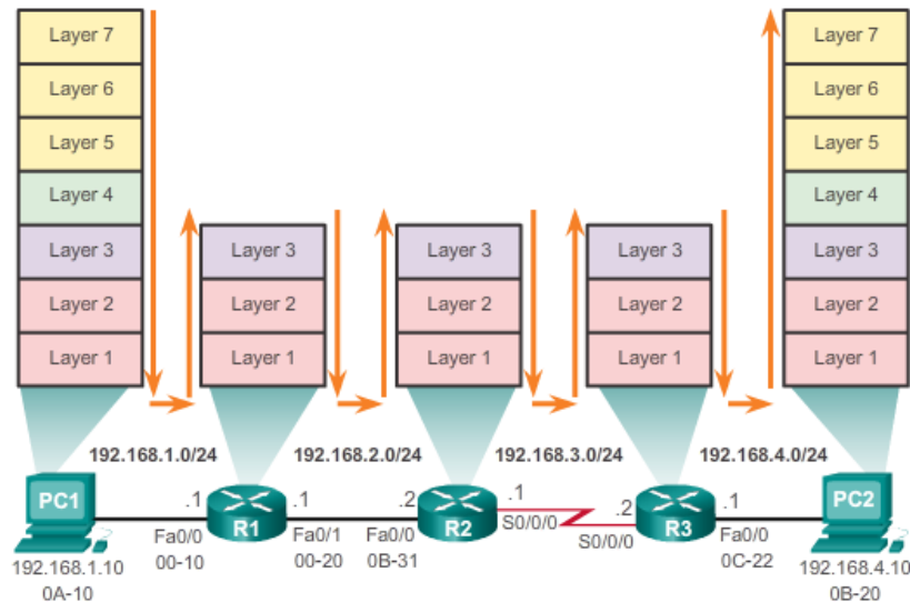
Fig. 4.13 Enkapsulasi dan De-enkapsulasi packet
