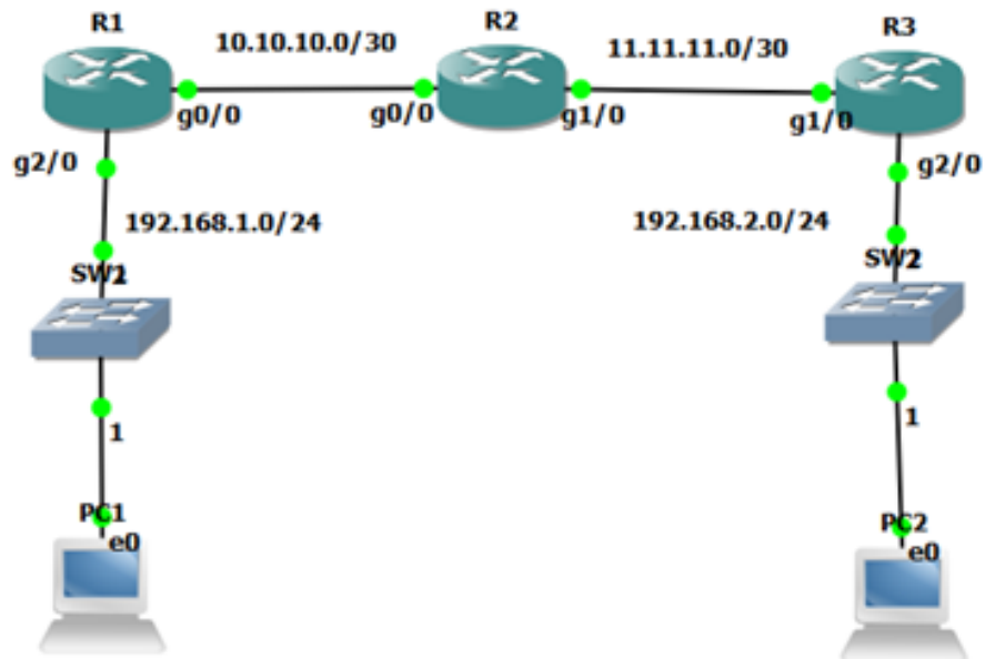
Fig. 7.16 Konfigurasi RIP
