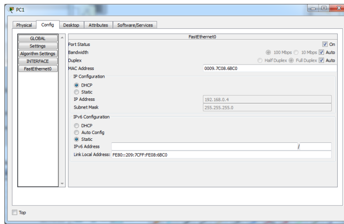
Fig. 10.4 Konfigurasi PC Client
