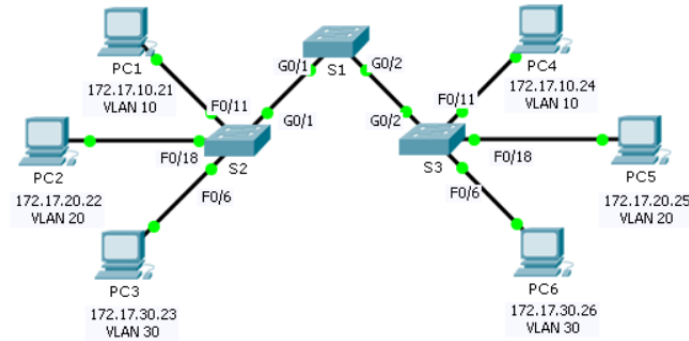
Fig. 3.13 Latihan Topologi
