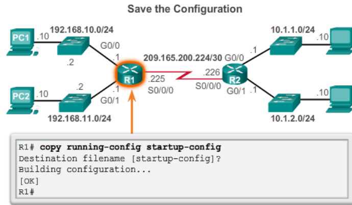
Fig. 4.8 Menyimpan konfigurasi
