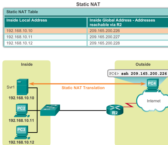
Fig. 11.2 Ilustrasi Statik NAT
