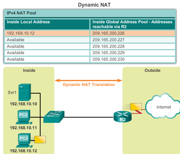
Fig. 11.3 Ilustrasi NAT Dinamis
