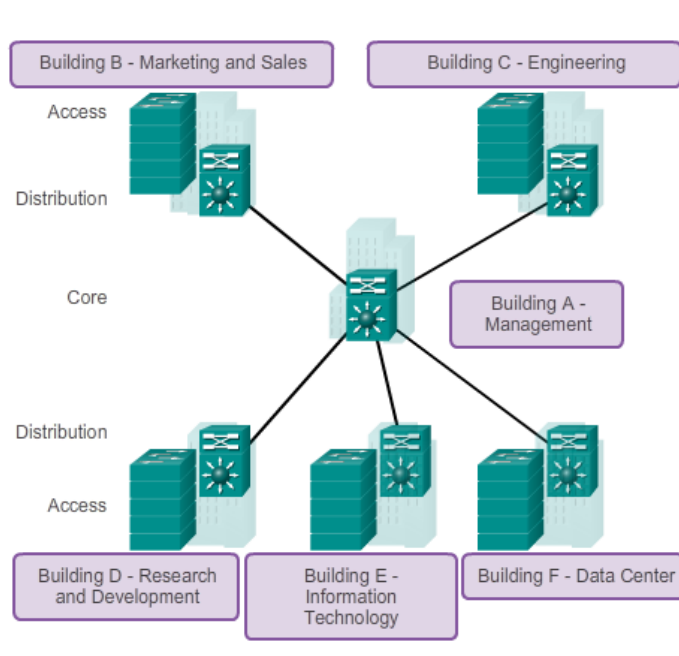
Fig. 1.7 Desain Jaringan Antar Gedung
