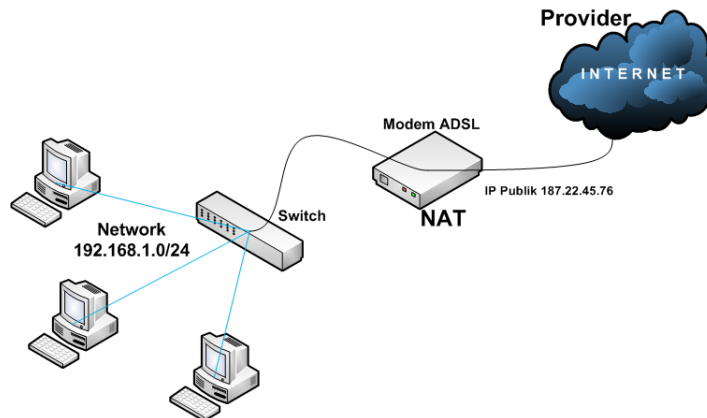
Fig. 11.1 Ilustrasi NAT
