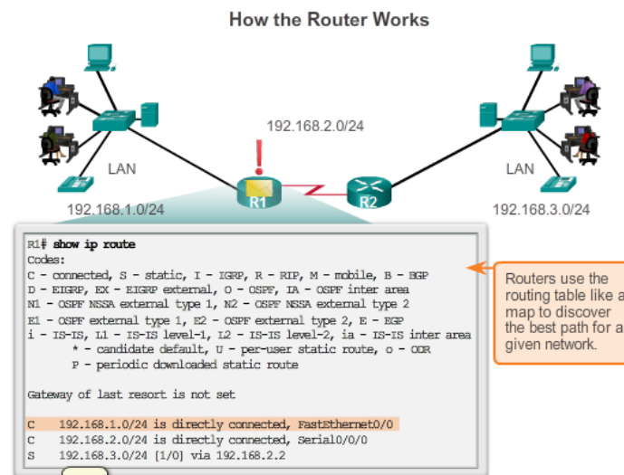
Fig. 4.3 Cara kerja routing
