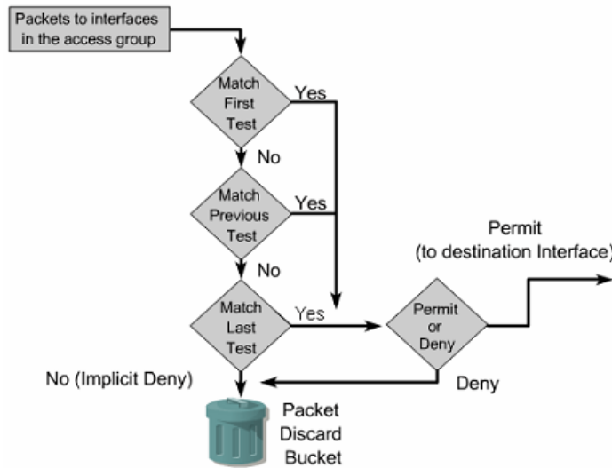
Fig. 9.2 Cara Kerja ACL
