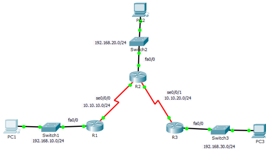
Fig. 8.3 Topologi OSPFv2
