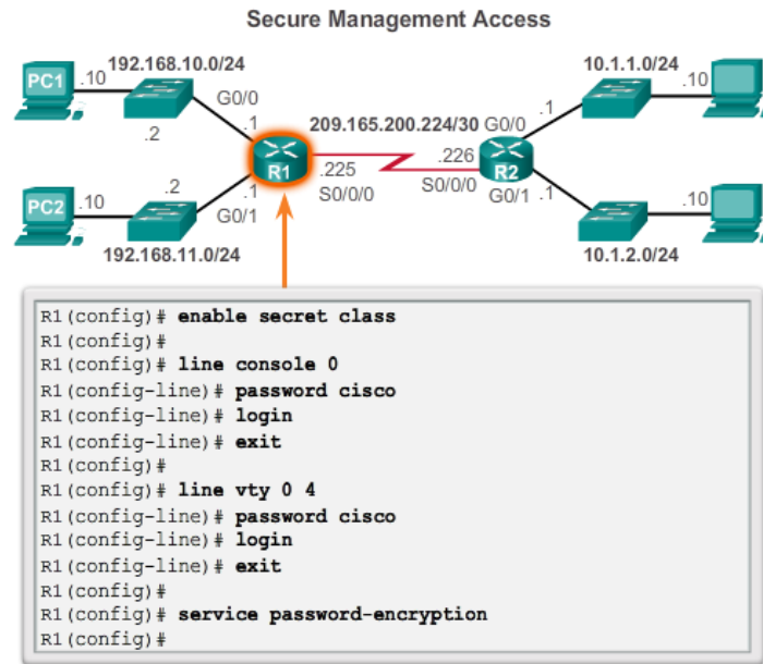
Fig. 4.6 Konfigurasi akses manajemen
