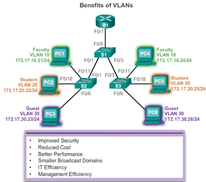
Fig. 3.1 Manfaat VLANs
