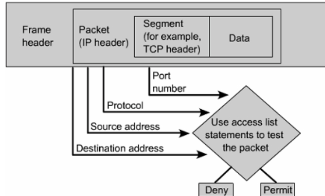
Fig. 9.1 Ilustrasi ACL
