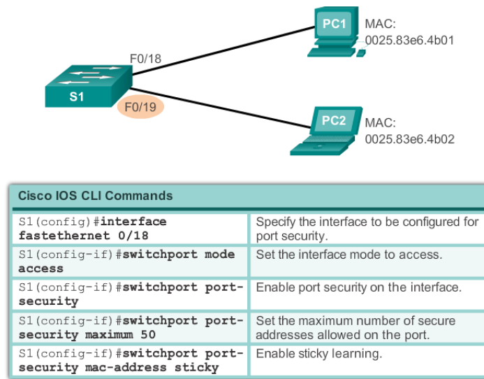
Fig. 2.11 Konfigurasi Sticky Port Security
