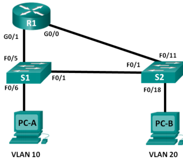
Fig. 5.4 Konfigurasi Router On A Stick
