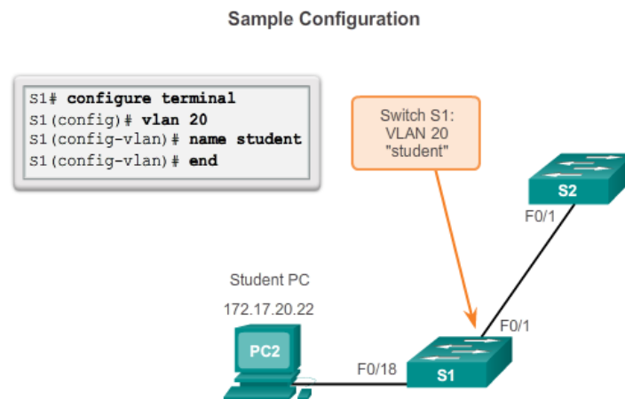
Fig. 3.7 Contoh Konfigurasi VLANs
