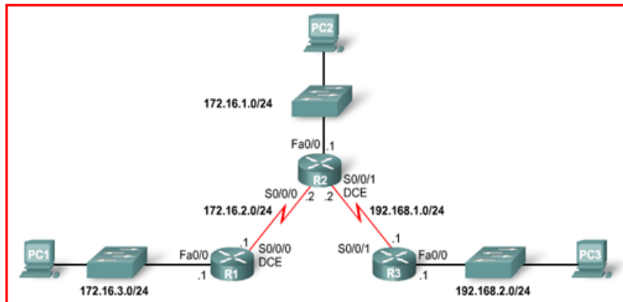
Fig. 6.5 Konfigurasi IPv4 Static Routing Pada Topology Jaringan
