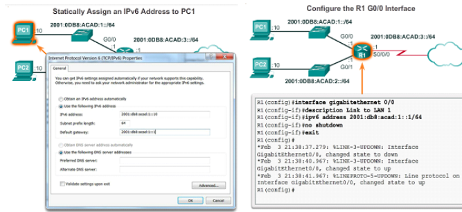
Fig. 4.10 Konfigurasi IPv6 router interface
