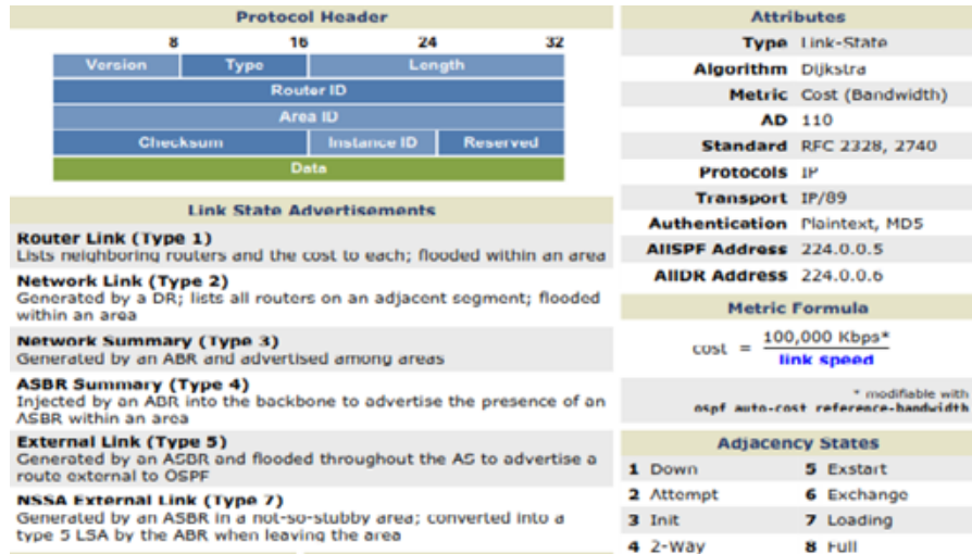
Fig. 7.19 OSPF Header
