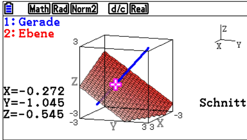
Schnittpunkt
