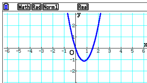
Grafikfenster
